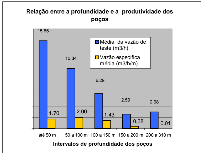
Figura 53 - Variação da produtividade dos poços com a profundidade.
