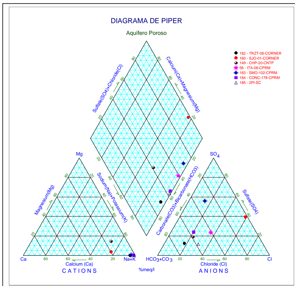
Figura 57 - Diagrama de Piper das amostras relativas aos aquíferos porosos.
