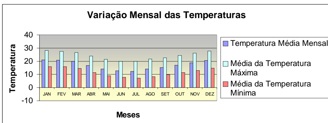
Figura 28 - Variação Mensal das Temperaturas na Estação Meteorológica de Xanxerê em 54 anos de observação.
