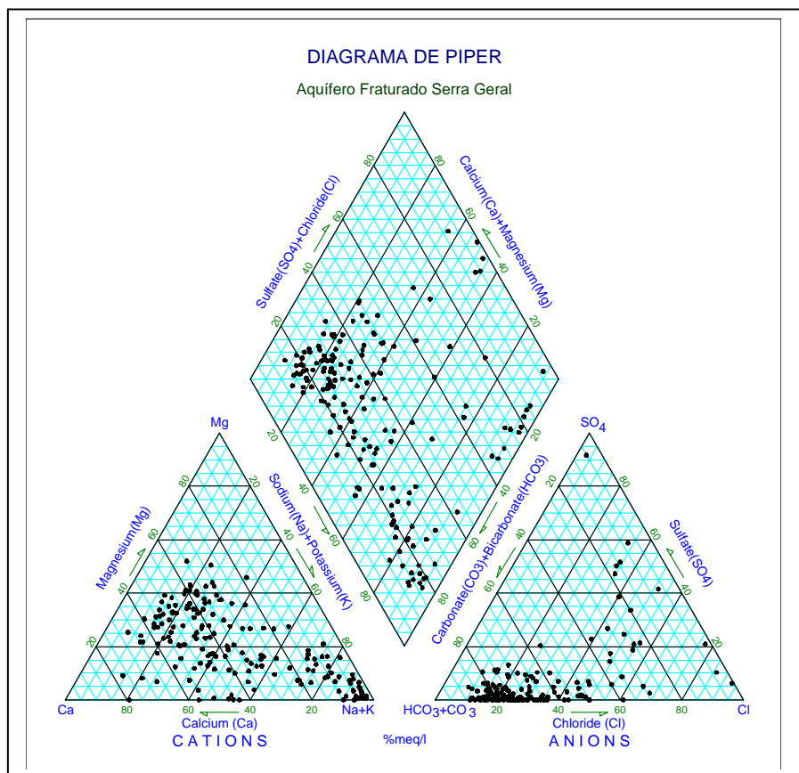
Figura 56 - Diagrama de Piper das amostras relativas aos aquíferos fraturados.
