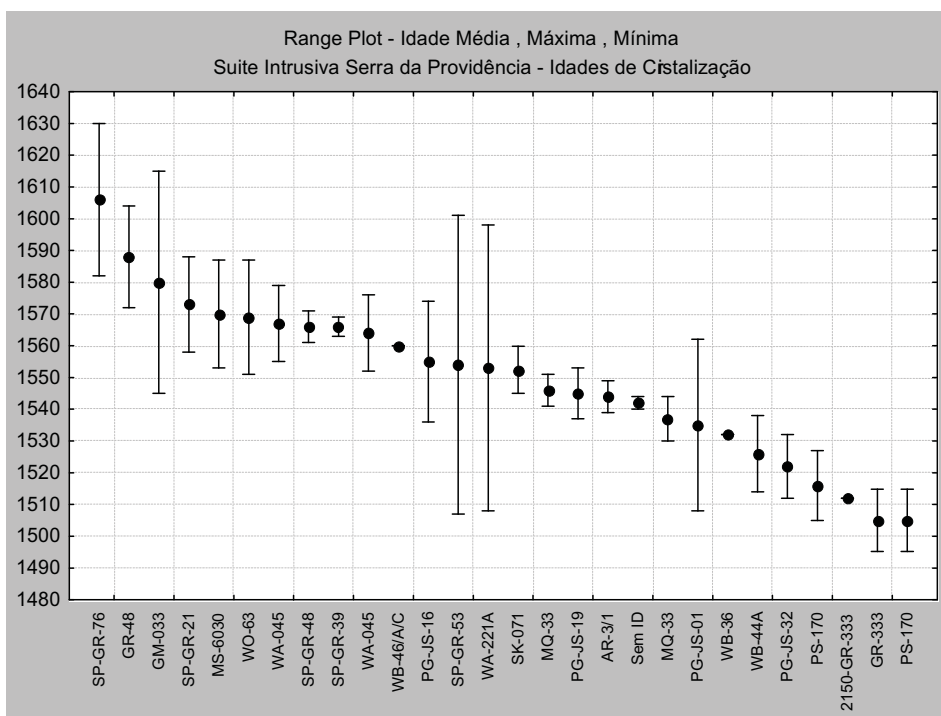
Figura 138 - Gráfico com as idades de cristalização e amplitude considerando o erro analítico.
