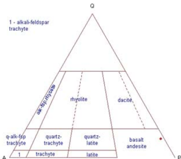
Figura 151 - Classificação modal da amostra PS-320. Streckeisen, (1976).
