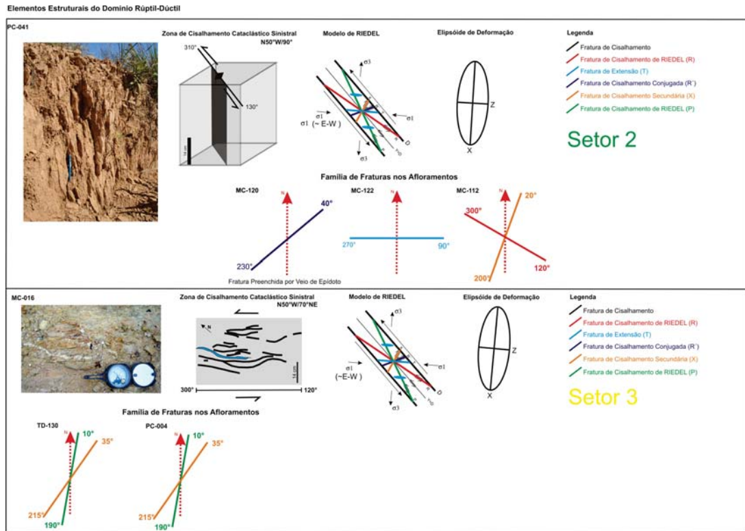
Figura 178 - Elementos Estruturais do Domínio Rúptil-Dúctil (Setores 2 e 3).
