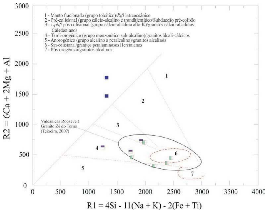
Figura 24 - Diagrama multicatiônico R1R2 adaptado por BATCHELOR e BOWDEN (1985) e usado na definição de ambientes tectônicos e sua relação com Suítes ígneas. Símbolos como Figura 21.
