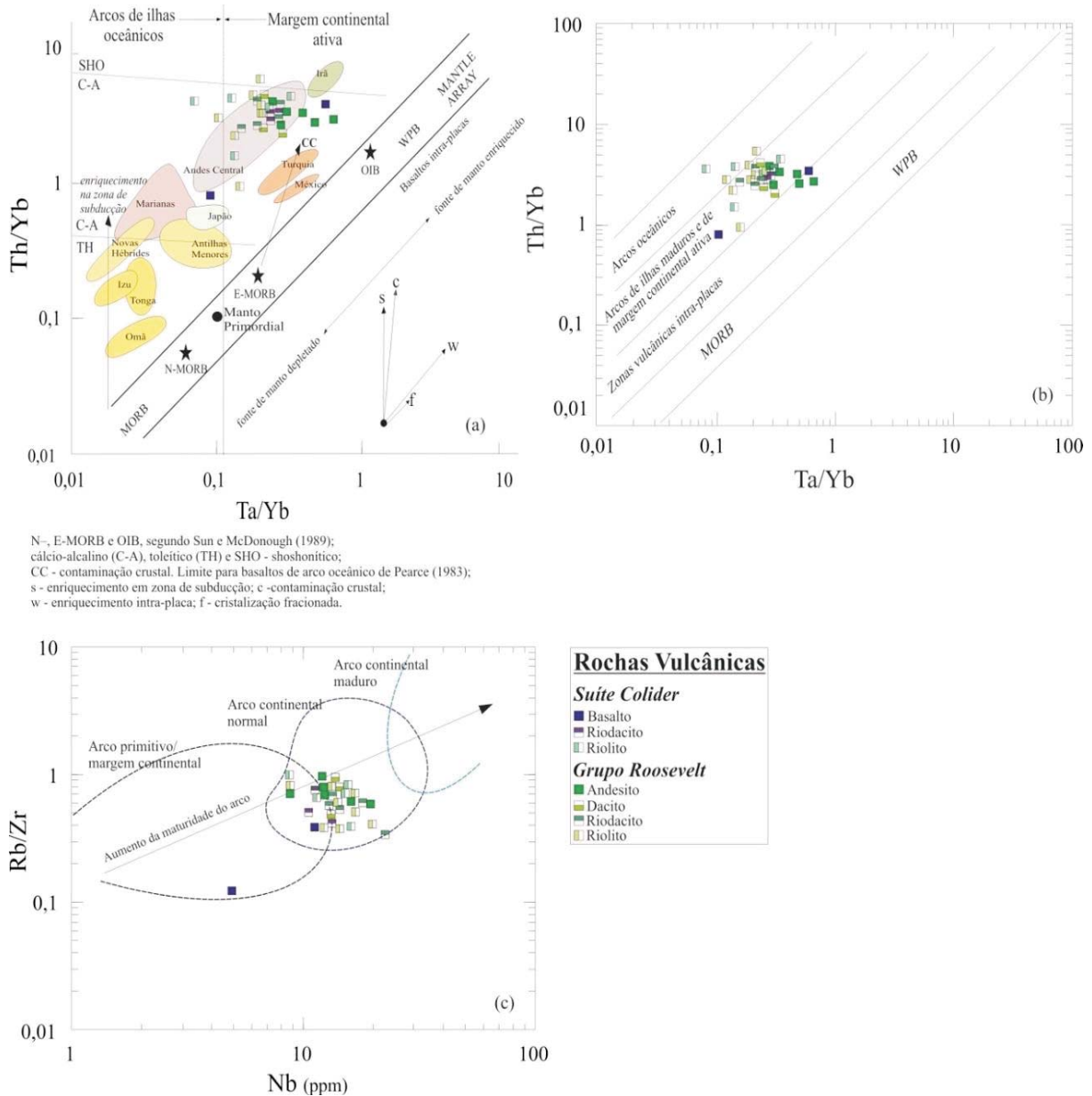
Figura 25 - Diagramas de caracterização de ambiente tectônico que utilizam razões de elementos-traço: em (a) PEARCE (1993), (b) SCHANDL e GORTON (2002) e em (c) BROWN et al., (1984).
