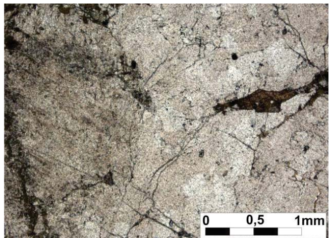
Fotomicrografia 72 - Plagioclásio saussuritizado e sericitizado (luz natural). Ponto PS 231.
