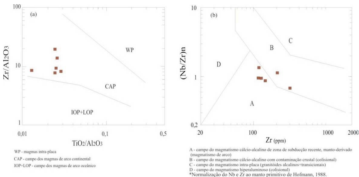
Figura 33 - Em (a) diagrama de MULLER et al., (1992) e CARR et al., (2003) e em (b) diagrama de THÍÉBLEMONT e TEGYÉY (1994) que ilustram a relação entre ambientes e fontes.
