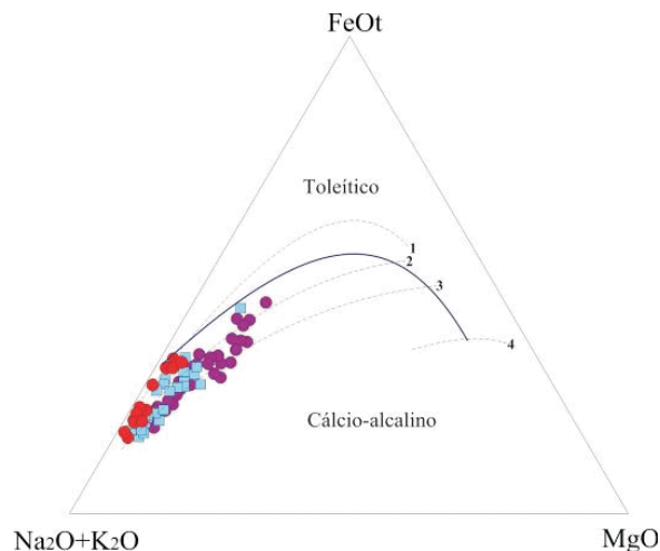
A linha sólida representa a divisão campo toleítico/cálcio-alcálico de Irvine e Baragar (1971), e as linhas tracejadas de 1 a 4 são vetores de aumento da maturidade do arco, segundo Brown (1982) e Knudsen e Andersen (1999). FeO como FeO T .
