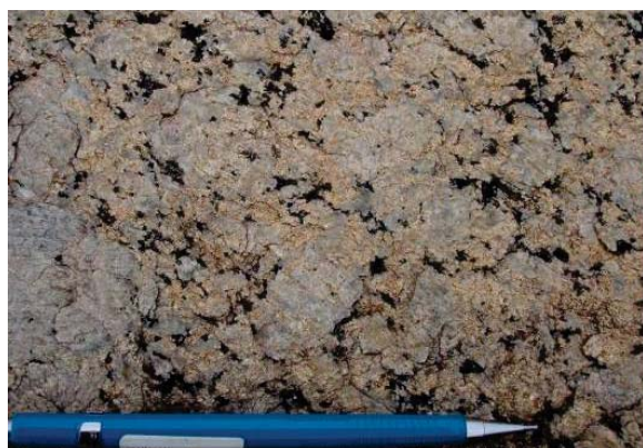
Foto 203 - Aspecto textural do granito da Suíte Intrusiva Serra da Providência.
