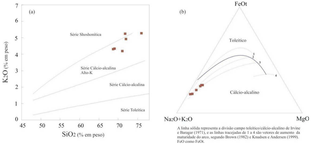
Figura 29 – Em (a) diagrama SiO_2 vs. K_2O de PECCERILLO E TAYLOR (1976) e a classificação dos granitos da Suíte Intrusiva Paranaíta como cálcio-alcálicos alto-K e em (b) diagrama AFM de IRVINE E BARAGAR (1971) e a confirmação do caráter cálcio-alcálico das amostras analisadas.
