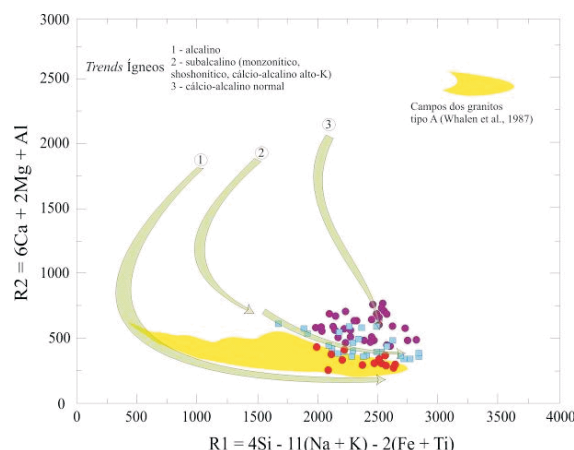
Figura 66 - Diagrama multicatiónico R1R2 usado para definir tendência ígnea (DeLaROCHE et al., 1980). Símbolos como Figura 60.
