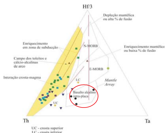
Figura 53 - Diagrama ternário Th vs. Hf/3 vs. Ta de WOOD (1980) e PEARCE e PEAT (1995) para as rochas máficas da área destacando-se o posicionamento intra-placas dos enclaves (simbolizados pelos círculos preenchidos na cor preta no interior do círculo vermelho). Símbolos como Figura 46.
