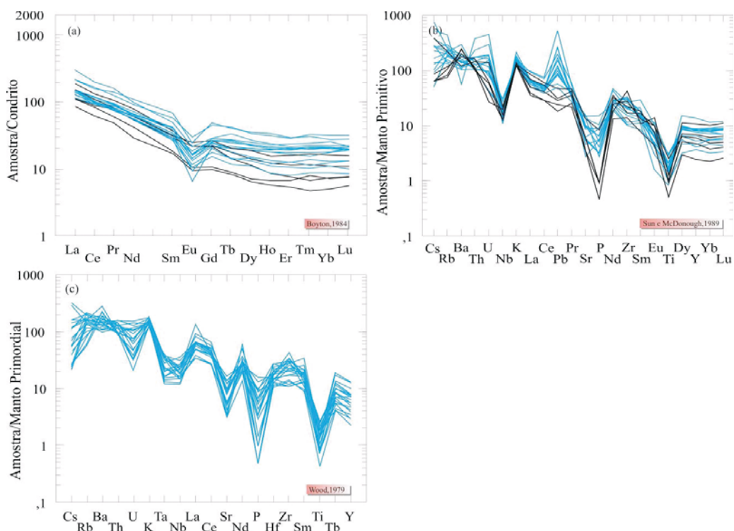
Figura 81 - Padrões de ETR (a) e spidergramas (b,c) dos sienogranitos e monzogranitos do Granito São Romão.
