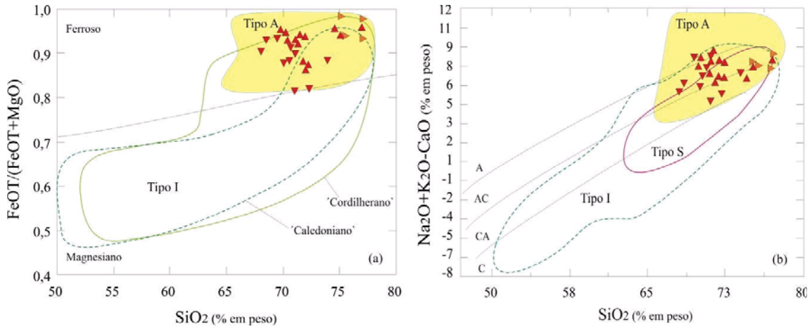
Figura 127 - Diagramas de FROST et. al.,(2001) que usam óxidos como discriminantes. Em (a) SiO_2 vs. FeOT/(FeOT+MgO) e (b) SiO_2 vs. Na_2O+K_2O-CaO (MALI). Símbolos como Figura 123.
