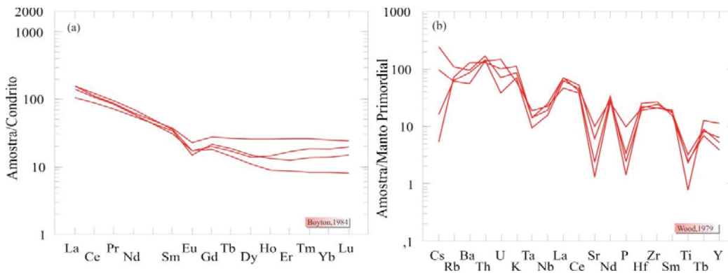
Figura 86 - Padrões de ETR dos granitos Apicás, em (a) normalizados ao condrito de BOYNTON (1984) e de multielementos normalizados ao manto primordial de WOOD (1979) em (b).
