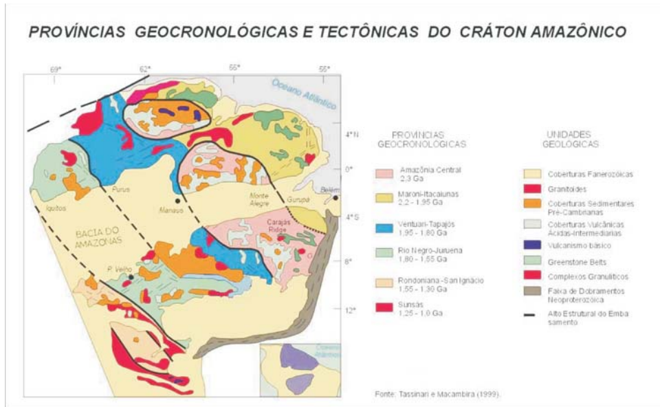
Figura 8 - Distribuição das províncias geocronológicas do Cráton Amazônico segundo TASSINARI E MACAMBIRA (1999).
