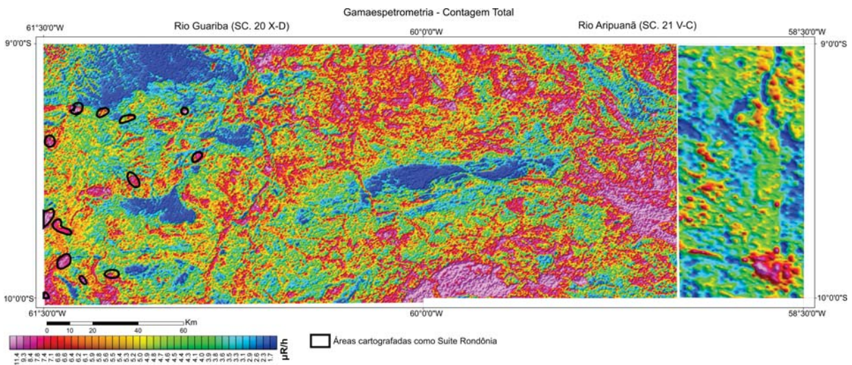
Figura 153 - Mapa gamaespectrométrico de contagem total, evidenciando os granitos da Suíte Intrusiva Rondônia na porção oeste da área.
