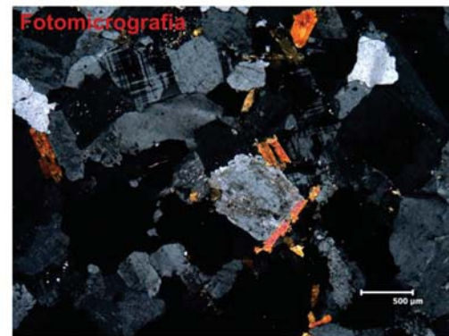
Cristais hipidiomórficos de feldspato, com quartzo intersticial e pequenas palhetas de biotita sem orientação preferencial.
