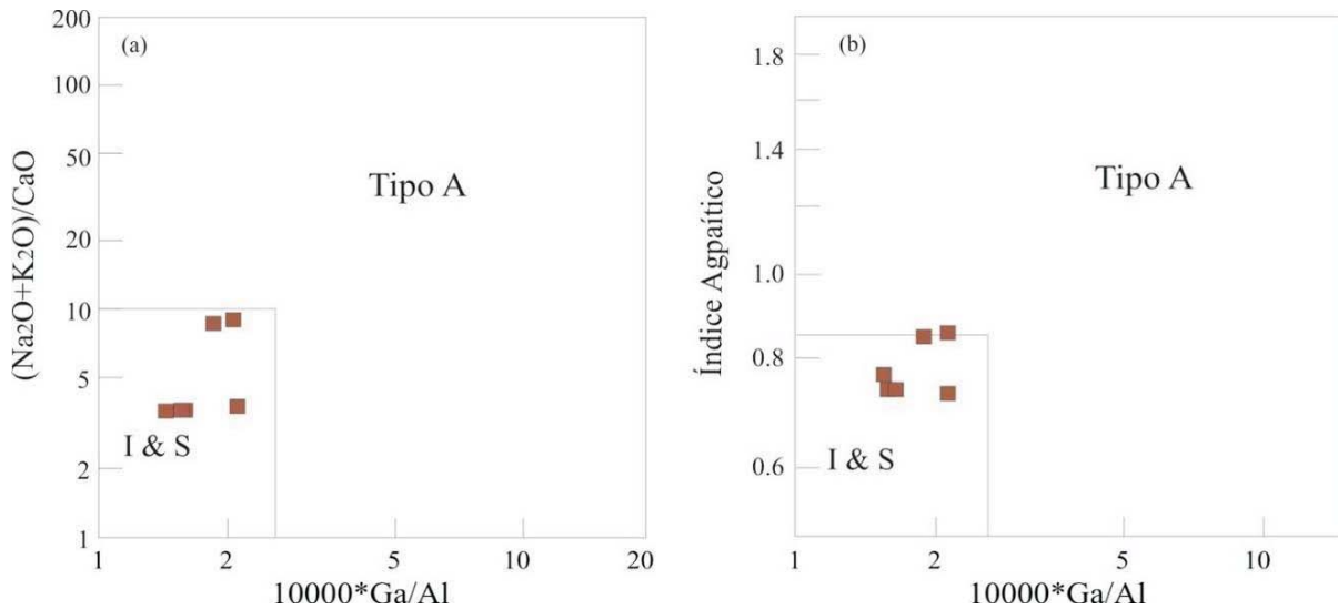
Figura 30 - Diagramas discriminantes de WHALEN et al., (1976) onde os granitos da Suíte Intrusiva Paranaíta caem no campo tipo I/S.
