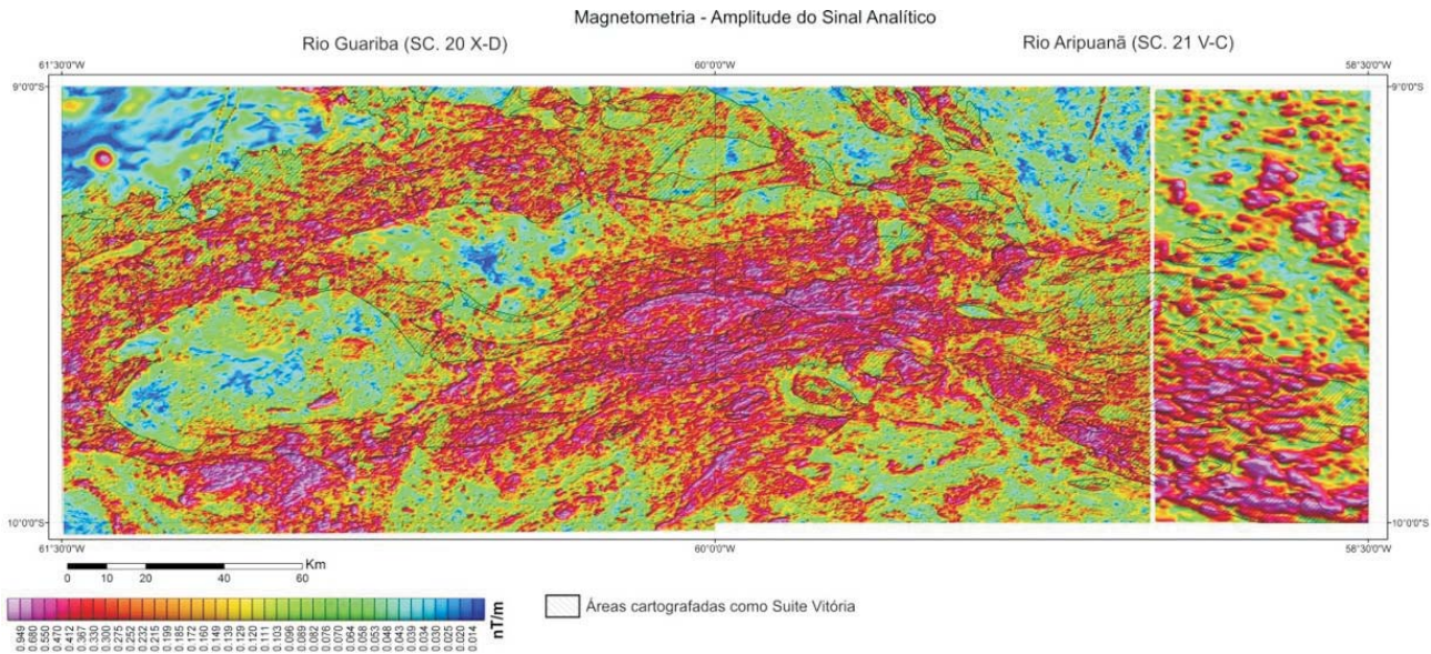
Figura 38 - Mapa aeromagnetométrico de amplitude do sinal analítico, evidenciando os contornos da Suíte Plutônica Vitória.
