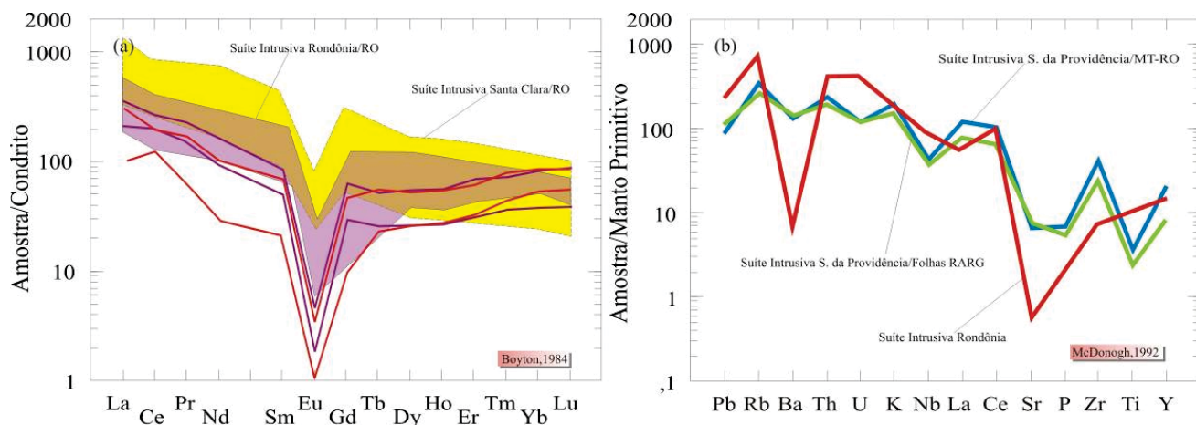
Figura 163 - Padrões de ETR dos granitos da Suíte Intrusiva Rondônia nas folhas Rio Aripuanã e Rio Guariba. (a) - Comparação com os granitos similares em Rondônia (BETTENCOURT et al., 1995) e em (b) diagrama de multielementos com a comparação dos padrões e das curvas médias com os granitos tipo A da Suíte Intrusiva Serra da Providência nas folhas Rio Aripuanã e Rio Guariba e em outras regiões do NW do Mato Grosso. Normalização ao Condrito de BOYNTON (1984) e ao Manto Primitivo de SUN e McDONOUGH (1989).
