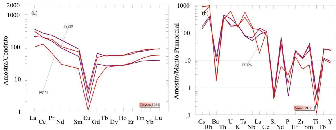
Figura 159 - Padrões de ETR (a) e de multielementos (b) dos sienogranitos da Suíte Intrusiva Rondônia. Normalização ao Condrito segundo BOYNTON (1984) e ao Manto Primordial de WOOD (1979).
