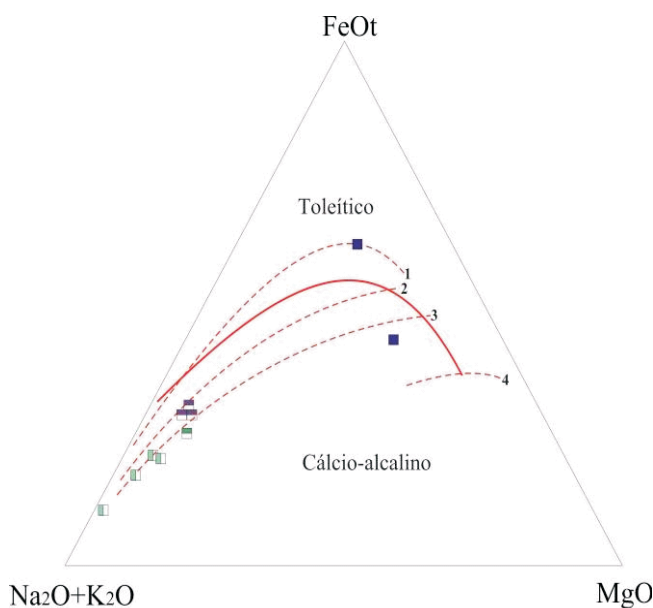
A linha sólida representa a divisão campo toleítico/cálcio-alcálico de Irvine e Baragar (1971), e as linhas tracejadas de 1 a 4 são vetores de aumento da maturidade do arco, segundo Brown (1982) e Knudsen e Andersen (1999). FeO como FeOt.
