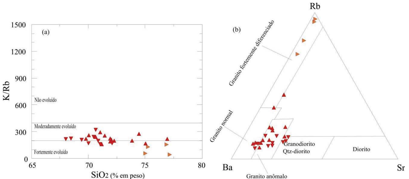
Figura 126 - Em (a) grau de evolução dos granitos estudados em termos da razão K/Rb e em (b) diagrama ternário preenchem os campos dos granitos anômalo e normais (ricos em Ba). Símbolos como na Figura 123.
