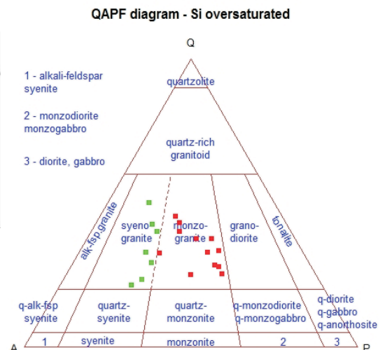
Figura 80 - Proporção dos constituintes mineralógicos principais das rochas do Granito São Romão e Diagrama QAP com a classificação modal. As informações foram compiladas de 19 análises petrográficas.
