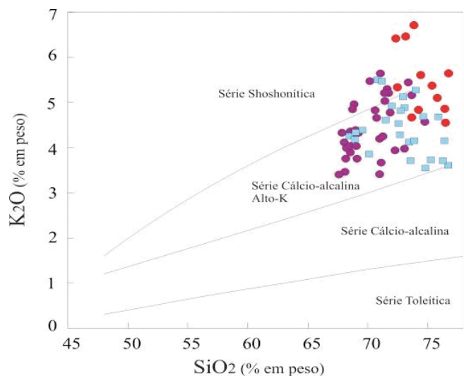
Figura 62 - Diagrama \text{SiO}_2 vs. \text{K}_2\text{O} de PECCERILLO E TAYLOR (1976) e a classificação dos granitos São Pedro como cálcio-alcinos alto a muito alto-K. Símbolos como Figura 60.
