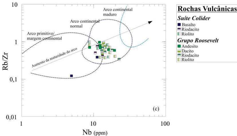
Figura 118 - Diagramas de caracterização de ambiente tectônico que utilizam razões de elementos-traço: em (a) PEARCE (1983), (b) SCHANDL e GORTON (2002) e em (c) BROWN et al., (1984).
