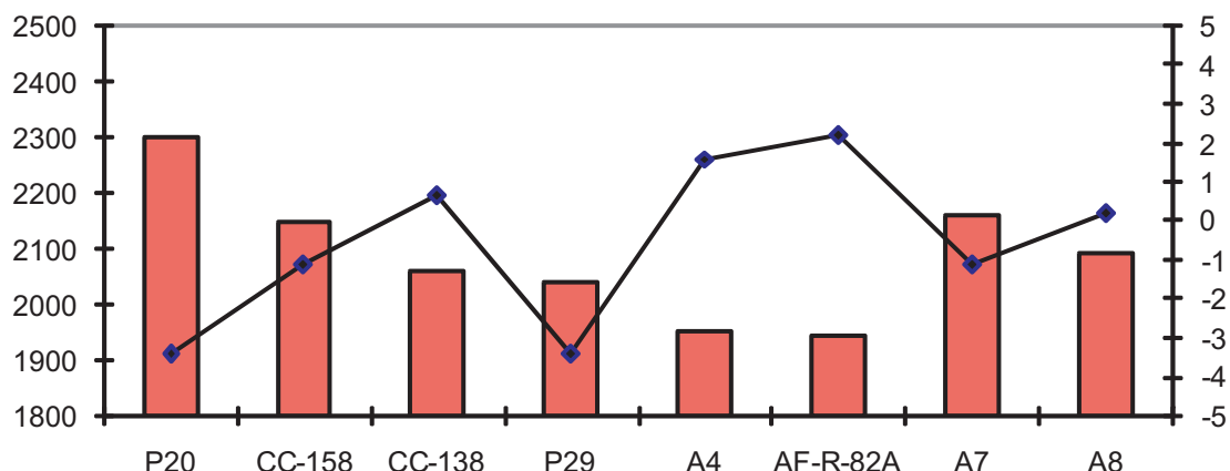
Figura 77 - Gráfico com as idades TDM Sm-Nd (eixo y esquerdo) e valores de εNd (eixo y direito)
