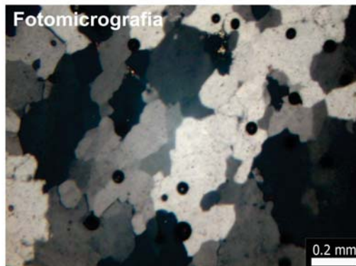
Cristais de quartzo apresentando extinção ondulante e bordas móveis.
