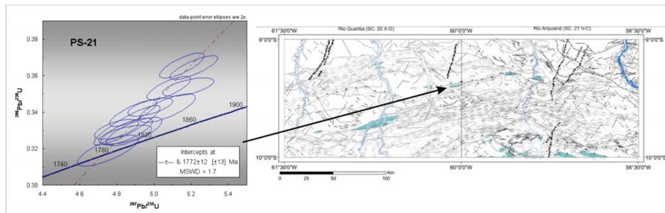
Figura 119 - Resultado da datação U-Pb TIMS realizada em zircão de metadacito, ponto PS-021.
