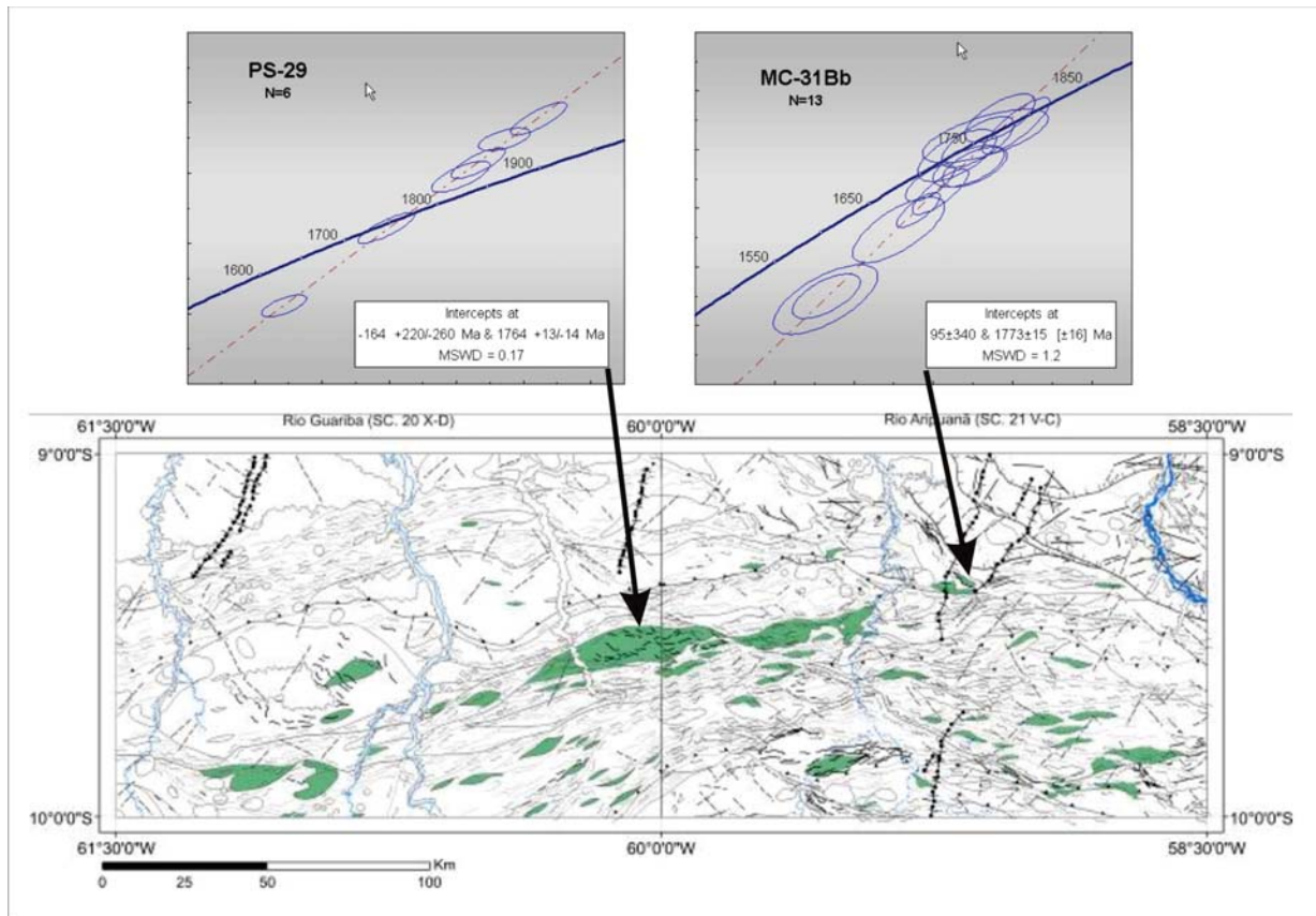
Figura 103 - Datações U-Pb e localização das amostras datadas. PS-029 UTM 822114/8942600 Zona 20S e MC-031Bb 283397/8939543 Zona 21S.
