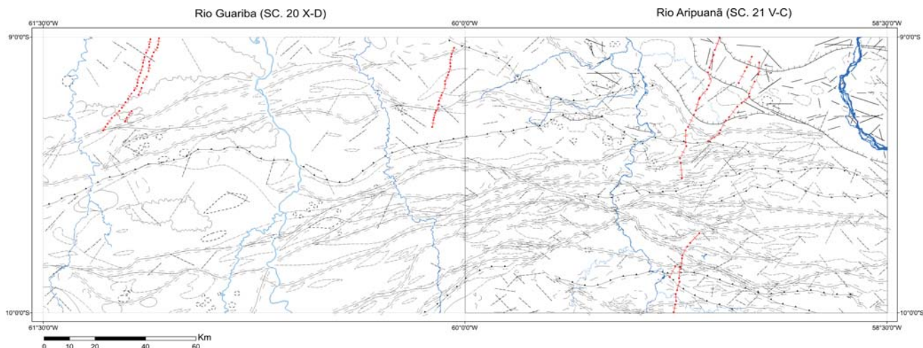
Figura 164 - Área de ocorrência dos principais diques mesozóicos (destacado em vermelho)
