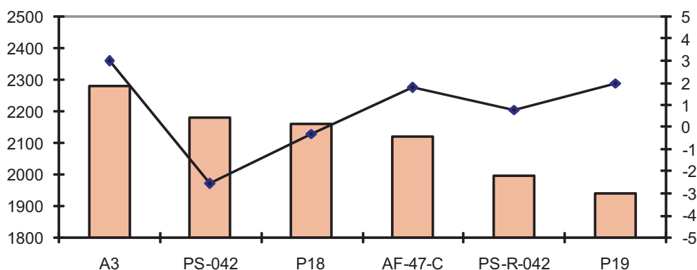
Figura 56 - Gráfico composto, com as idades T_{DM} Sm-Nd (eixo y esquerdo) e valores de \epsilon_{Nd} (eixo y, à direita).
