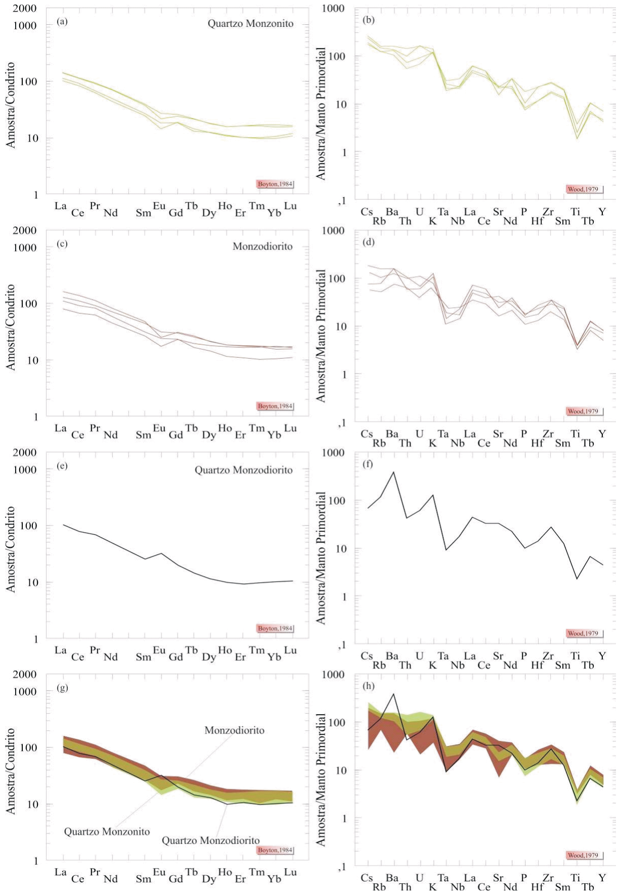
Figura 49 - Padrões de ETR e de multielementos dos monzodioritos, quartzo monzonitos e quartzo monzodiorito da Suíte Plutônica Vitória. Normalização ao condrito de BOYNTON (1984) e manto primordial de WOOD (1979). Nas Figuras g,h envelopes e curvas comparativas dos três tipos de rocha.
