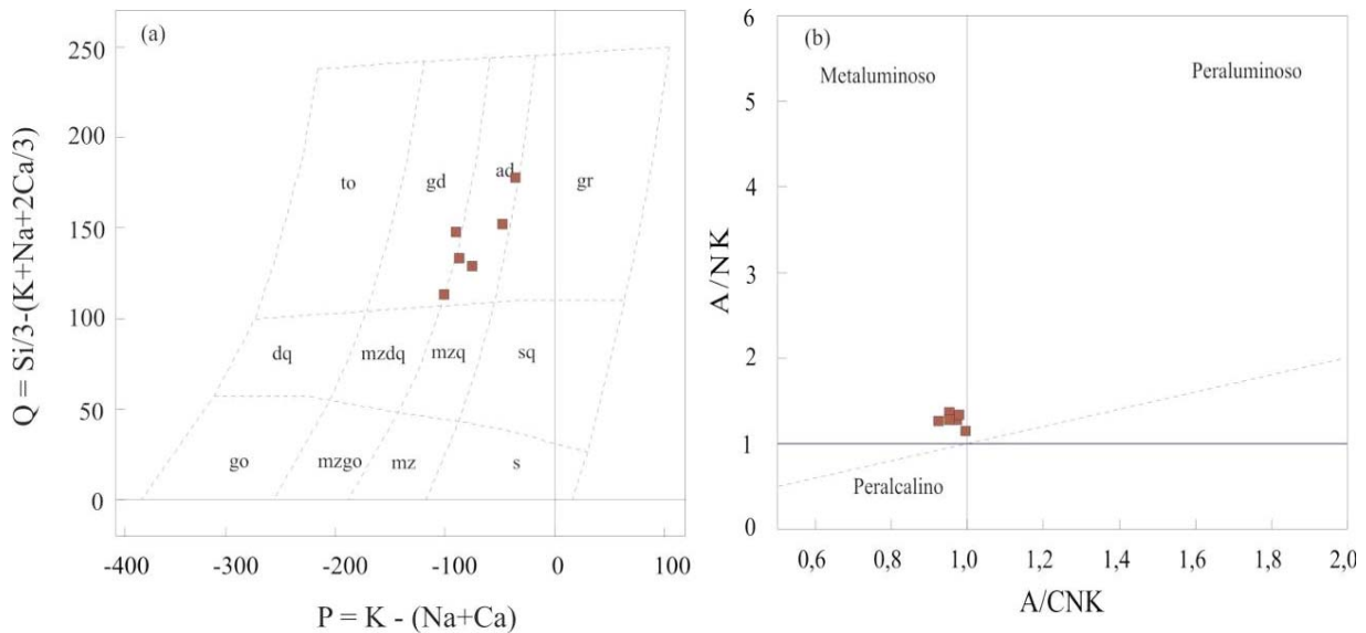
Figura 28 -- Em (a) diagrama de classificação química de granitóides de DEBON e LeFORT (1983) e em (b) diagrama de classificação para os granitos Paranaíta a partir da razão molecular ANK vs. ACNK (MANIAR e PICCOLI, 1989).
