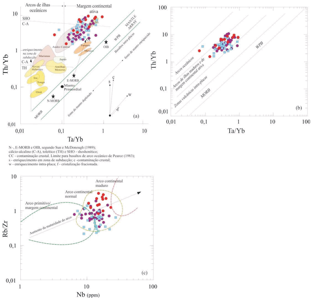
Figura 74 - Diagramas de caracterização de ambiente tectônico que utilizam razões de elementos-traço: em (a) PEARCE (1983), (b) SCHANDL e GORTON (2002) e em (c) BROWN et al. (1984). Símbolos como Figura 60.
