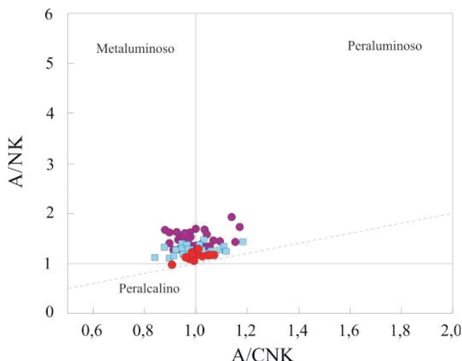
Figura 63 - Diagrama de classificação para os granitos São Pedro a partir da razão molecular ANK vs. ACNK (MANIAR e PICCOLI, 1989). Símbolos como Figura 60.
