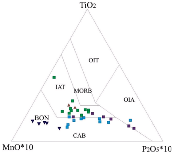
Figura 96 - Diagrama ternário de MULLEN (1983) que usa óxidos para definir composição das rochas de arco. OIT – toleítos de ilhas oceânicas; IAT – toleítos de arco de ilhas; MORB – basaltos de dorsais meso-oceânicas; OIA – alcálicas de ilhas oceânicas; CAB – basaltos cálcio-alcálicos e BOM – boninitos. Símbolos como Figura 95.
