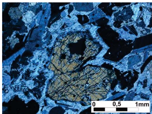
Fotomicrografia 54 - Textura coronítica no Cpx com bordas de plagioclásio, por vezes com textura simplectítica (exsoluções de opacos) em metandesito (luz polarizada). Ponto PS-206.
