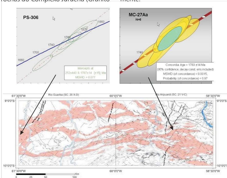
Figura 55 - Resultados analíticos U-Pb e localização das amostras de metagranodiorito e metatonalito do Suíte Plutônica Vitória. PS - 306 (UTM Z 20S- 684380/8954472) e MC- 27Aa (UTM Z 21S- 265686/8958090).
