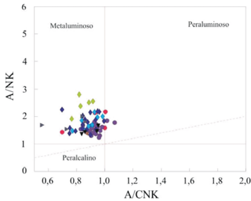
Figura 43 - Diagrama de classificação para as rochas intermediárias do Suíte Plutônica Vitória a partir da razão molecular ANK vs. ACNK (MANIAR e PICCOLI, 1989). Símbolos como Figura 40.
