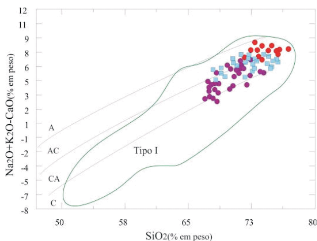
Figura 65 - Diagrama Na2O+K2O-CaO (MALI) vs. SiO2 de FROST et al., (2001) e os granitos São Pedro. Símbolos como Figura 60.
