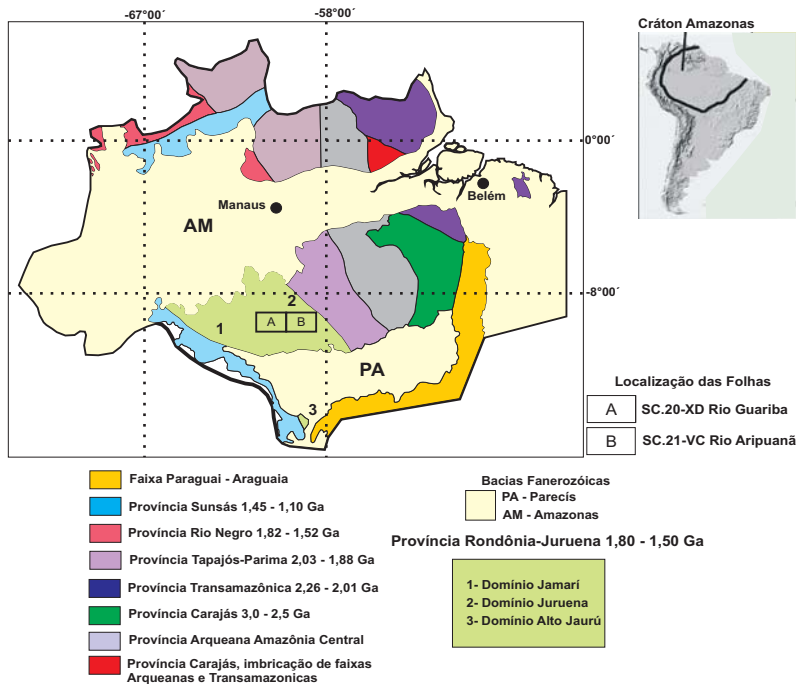
Figura 9 - Províncias Geocronológicas do Cráton Amazônico segundo SANTOS et al. , 2008 (modificada) e a localização das áreas mapeadas.
