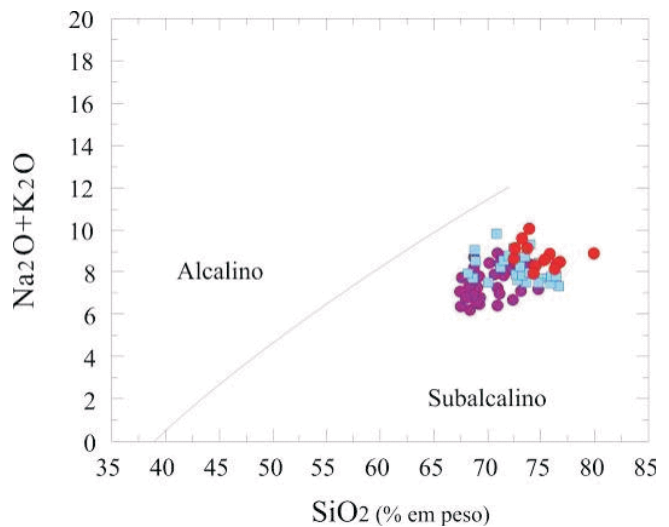
Figura 61 - Diagrama sílica vs. álcalis (TAS) de IRVINE E BARAGAR (1971). Símbolos como Figura 60.
