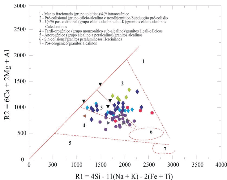
Figura 51 - Diagrama multicatiônico R1/R2 adaptado por BATCHELOR e BOWDEN (1985) usado na definição de ambientes tectônicos e sua relação com Suítes ígneas. Símbolos como Figura 46.
