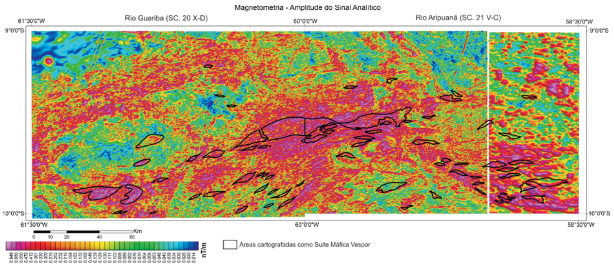
Figura 91 - Mapa magnetométrico de sinal analítico evidenciando os principais corpos da Suíte Máfica Vespore.
