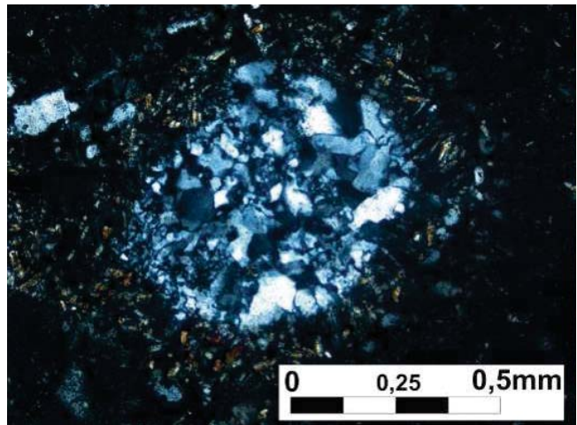
Fotomicrografia 65 - Cristais de quartzo preenchendo amídalas, bordejado por cristais prismáticos de epidoto (luz polarizada). Ponto PS-320.
