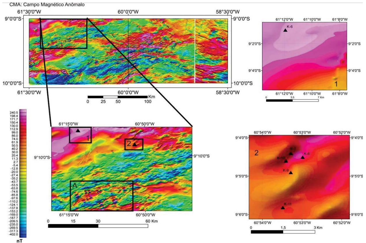
Figura 228 - Mapa aerogeofísico de campo magnético anômalo das folhas Rio Guariba e Rio Aripuanã, evidenciando as áreas de ocorrência dos corpos kimberlíticos (Áreas 1 e 2) e dipolos magnéticos (Área A).
