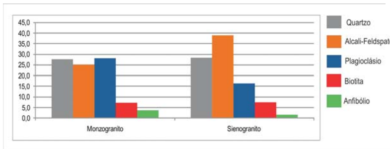
Figura 80 - Proporção dos constituintes mineralógicos principais das rochas do Granito São Romão e Diagrama QAP com a classificação modal. As informações foram compiladas de 19 análises petrográficas.
