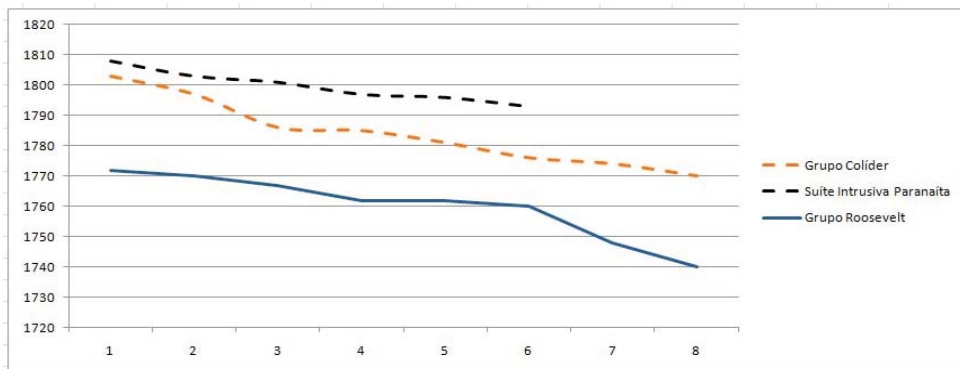
Figura 26 - Resultados das análises U-Pb apresentados na forma de gráfico.
