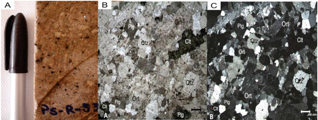
Figura 215 - A: Amostra de testemunho de sondagem do sienogranito encaixante, hidrotermalizado B: Plagioclásio (Plg) e ortoclásio (Ort) turvos, argilizados/ sericitizados e quartzo (Qtz), além de pseudomorfos de clorita (Clt) configurando textura inequigranular subidiomórfica fina a média (luz natural); C: luz polarizada. Ponto PS-531.
