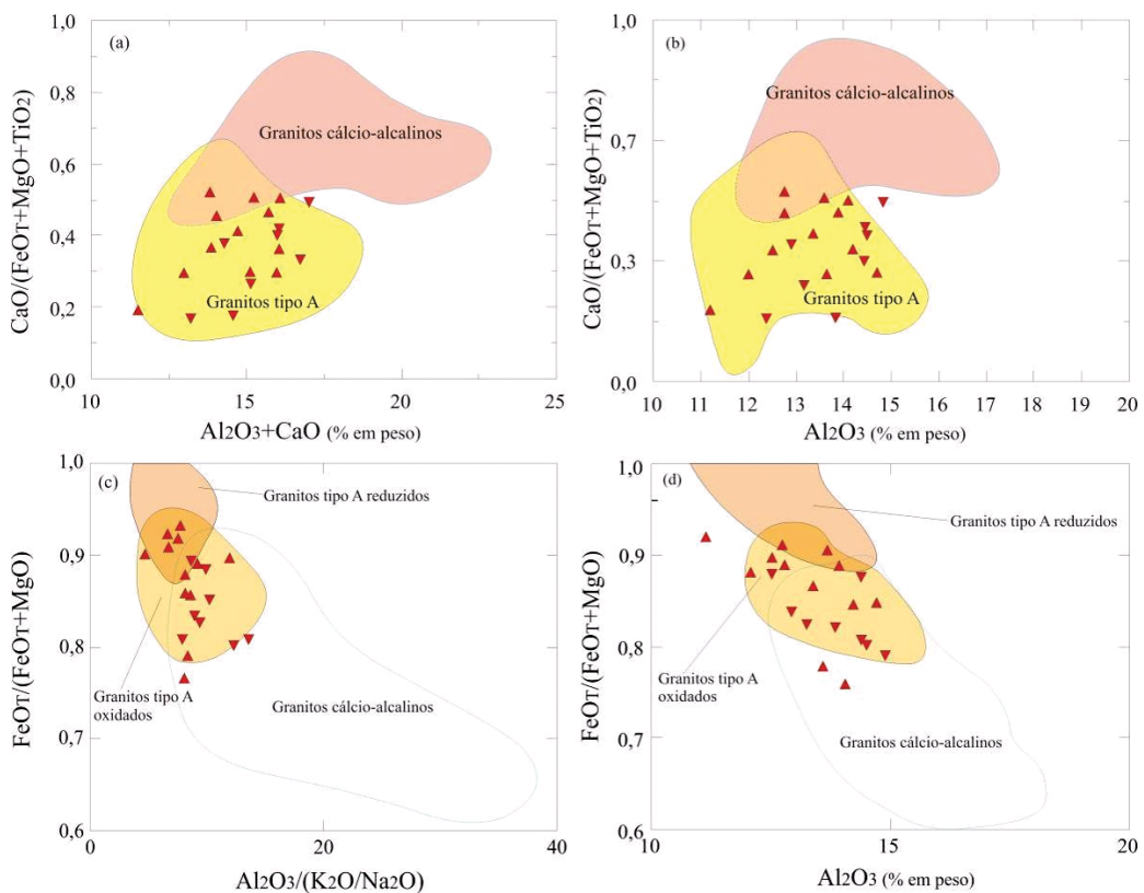
Figura 128 - Diagramas discriminantes que usam óxidos para a separação entre granitóides dos tipos I e A oxidados e reduzidos (DALL´AGNOLL e OLIVEIRA, 2007). Símbolos como Figura 123.
