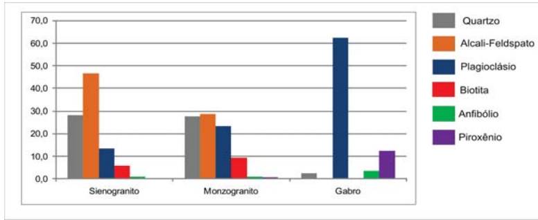
Figura 122 - Distribuição média dos minerais essenciais das rochas da Suíte Serra da Providência (a esquerda) e Classificação dos granitos e gabros da Suíte Intrusiva Serra da Providência segundo Streckeisen, (1976) (a direita)
