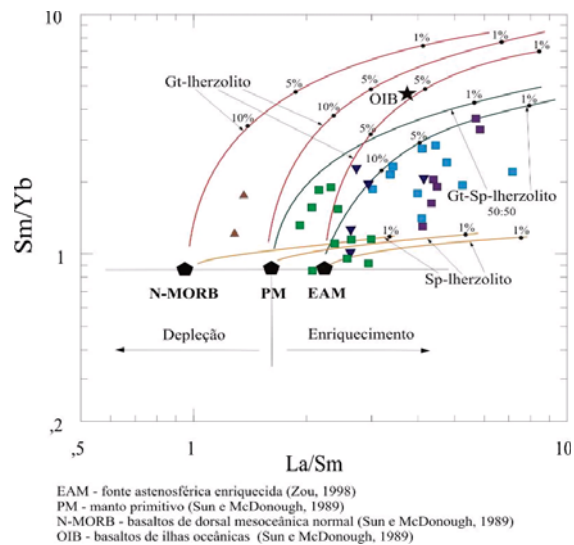
Figura 102 - Diagrama log Sm/Yb vs. log La/Sm mostrando as curvas de fusão obtidas usando-se a equação de fusão não-modal de SHAW (1970) através de método proposto por ALBAREDE (1998). Curvas de fusão para manto espinélio lherzolítico e granada lherzolítico. Coeficientes de partição mineral-matriz de McKENZIE e O'NIONS (1991). Símbolos como Figura 95.
