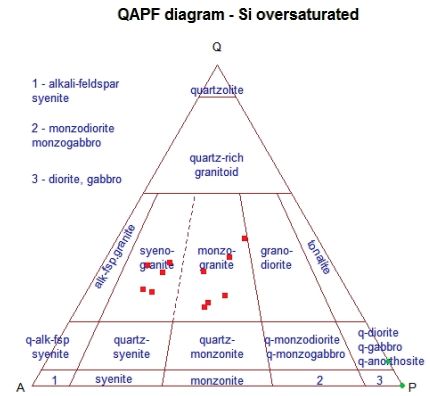
Figura 122 - Distribuição média dos minerais essenciais das rochas da Suíte Serra da Providência (a esquerda) e Classificação dos granitos e gabros da Suíte Intrusiva Serra da Providência segundo Streckeisen, (1976) (a direita)
