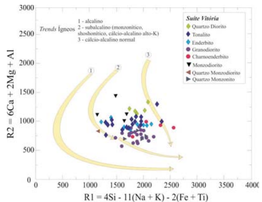
Figura 46 - Diagrama multicatiônico R1/R2 usado para definir tendência ígnea da associação de rochas do Suíte Plutônica Vitória (DeLaROCHE et al., 1980).
