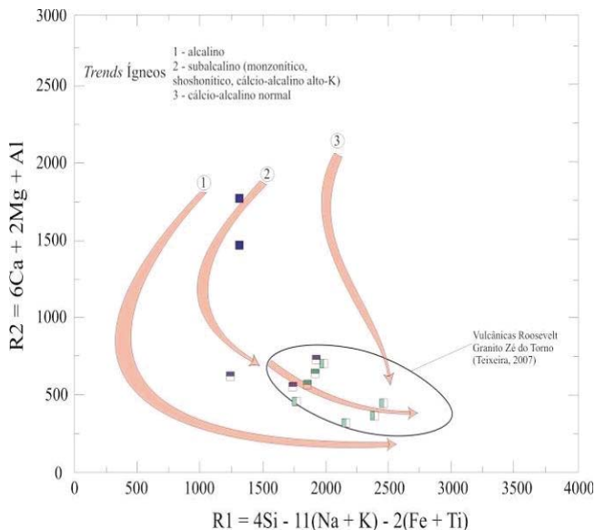
Figura 18 - Diagrama multicatiônico R1R2 usado para definir a tendência ígnea das rochas vulcânicas do Grupo Colíder nas folhas Rio Aripuanã e Rio Guariba de DeLaROCHE et al. (1980). Símbolos como Figura 14.
