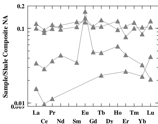
Figura 4.7: padrão dos ETRs dos mármorees da sub-unidade Guia normalizado ao folhelho NASC de Haskin et al. (1968).
