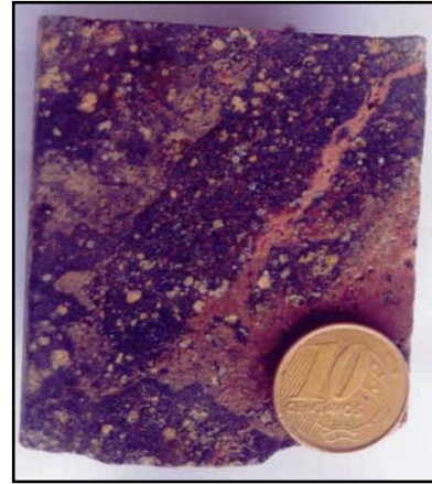
Figura 6.14: Brecha carbonosa constituída de fragmentos de rocha feldspática, colofanito, mármore e calcissilicática em matriz cinza escura de grafita e matéria orgânica amorfa.
