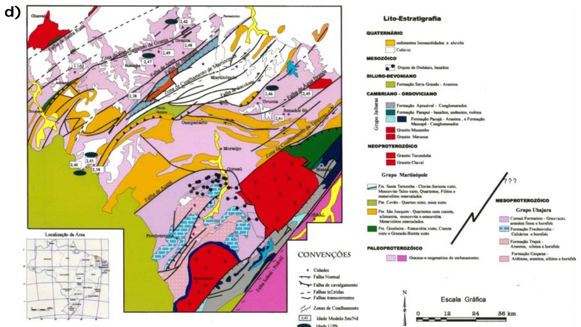
Figura 2.4: Geologia dos domínios da Província Borborema Setentrional – a) Maciço São José do Campestre (Dantas, 1998); b) Faixa Seridó e Maciço Rio Piranha (Dantas et al., 2003); c) Maciço Rio Piranha e Domínio Orós Jaguaribe (Cavalcante, 1999); d) Noroeste Ceará (Santos, 1999).
