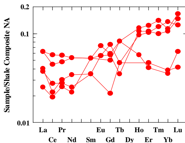
Figura 4.8: padrão dos ETRs dos mármorees da área normalizado ao folhelho NASC de Haskin et al. (1968).
