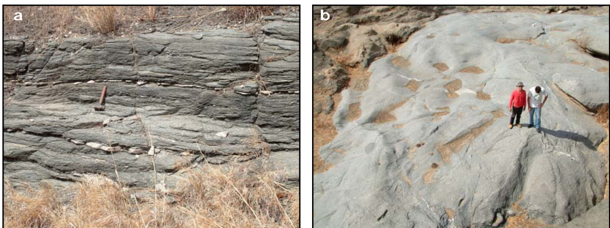
Figura 5.3: Afloramento pouco deformado dos metatonalitos da Suíte Madalena (a) e detalhe de a (b) (434839/9461658).
