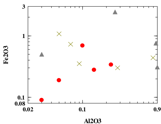
Figura 4.4: Diagrama Fe 2 O 3 -Al 2 O 3 dos mármoreis da área. Os símbolos são os mesmos da figura 4.3.
