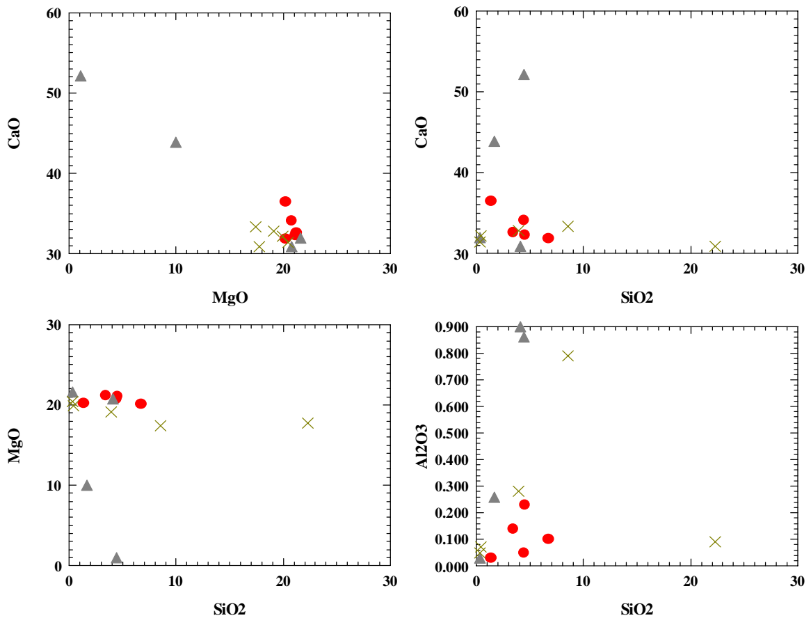
Figura 4.3: Relações entre os principais elementos maiores encontrados juntos aos mármoreis. A- Diagrama CaO-MgO; B- Diagrama CaO -SiO 2 ; C- Diagrama MgO-SiO 2 ; D- Al 2 O 3 -SiO 2 . Os símbolos em cruz representam os mármoreis da Folha Quixeramobim, os círculos em vermelhos os mármoreis da Folha Boa Viagem e os triângulos os mármoreis da Folha Itatira.
