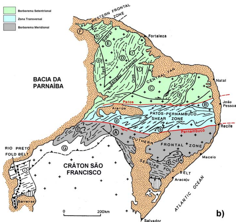
Figura 2.1b: Subdivisão da Província Borborema (Trompette, 1994).
