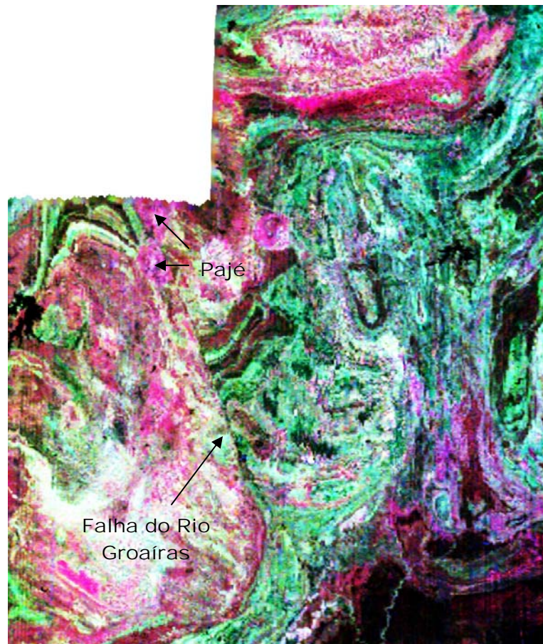
Figura 5.22: Deslocamento aparente do granito do Pajé pela falha do Rio Groaíras (Composição colorida RGB K:Th:U - Projeto Itatira/NUCLEBRÁS).
