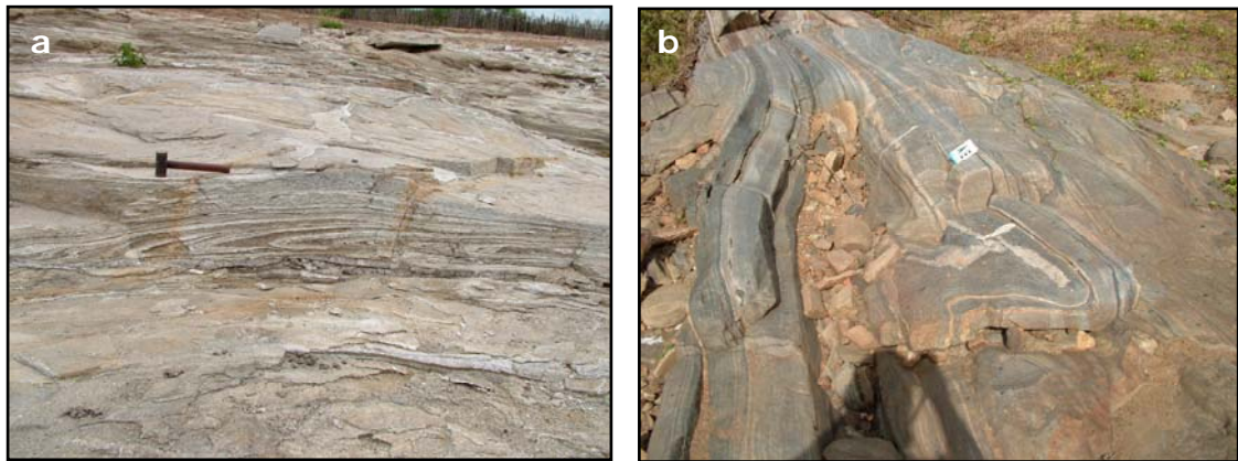
Figura 5.2: Dobra intrafolia associada a uma transposição (a) e dobramento do bandamento nos gnaisses do Complexo Cruzeta (b) (448409/9425560; 426966/9440982).
