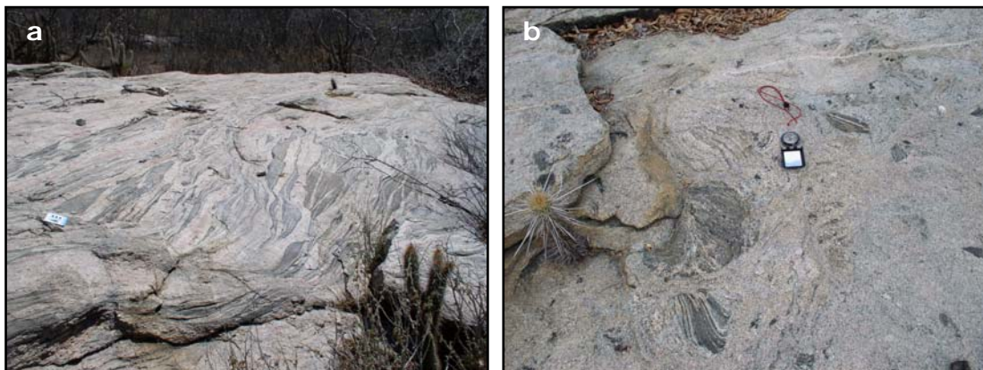
Figura 5.16: Exemplos de migmatização em condições dinâmicas (a) e estáticas (b) no Complexo Tamboril-Santa Quitéria.
